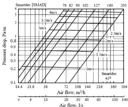
Perte de charge 45°
