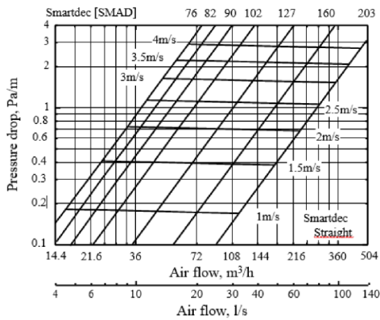
Druckverlust Gerade Länge
