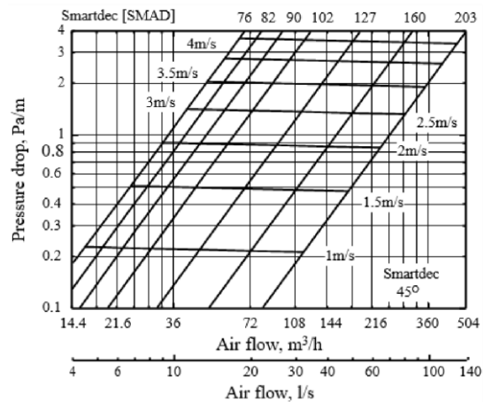
Druckverlust 45°
