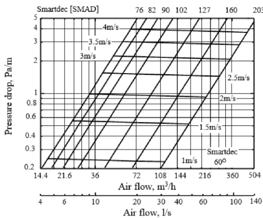
Druckverlust 60°
