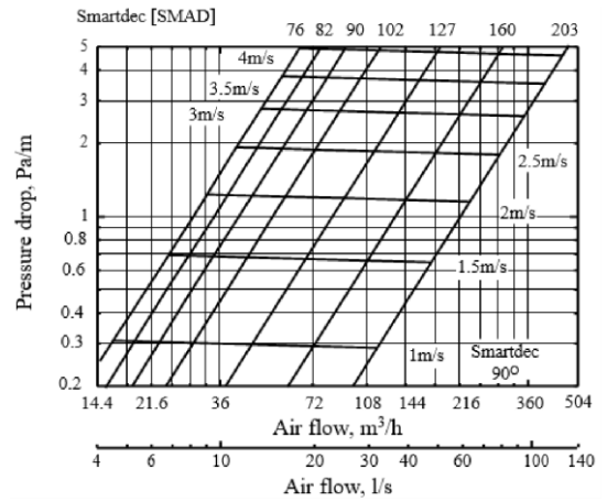
Druckverlust 90°
